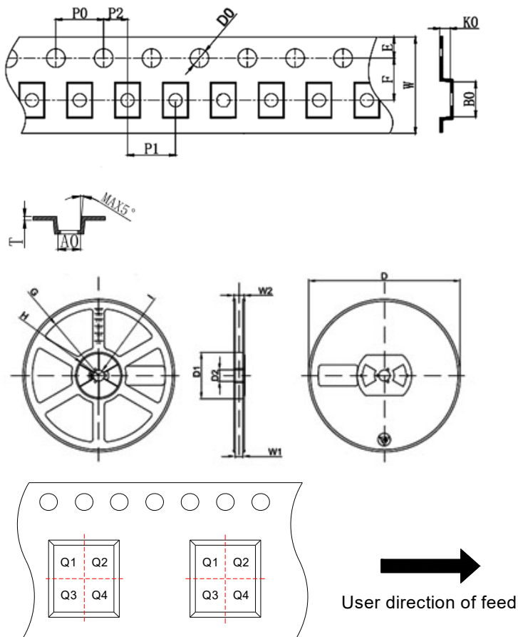
Pin 1 quadrant:Q1&Q2
