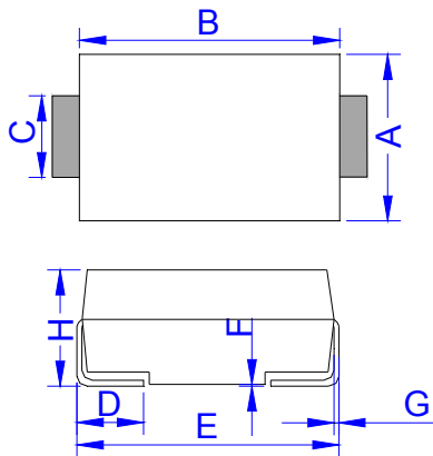
DO-214AC (SMA)
